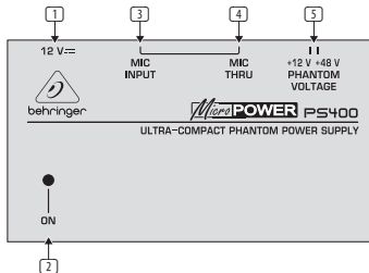
Bild 1: PS400-kontakter och kontrollelement
